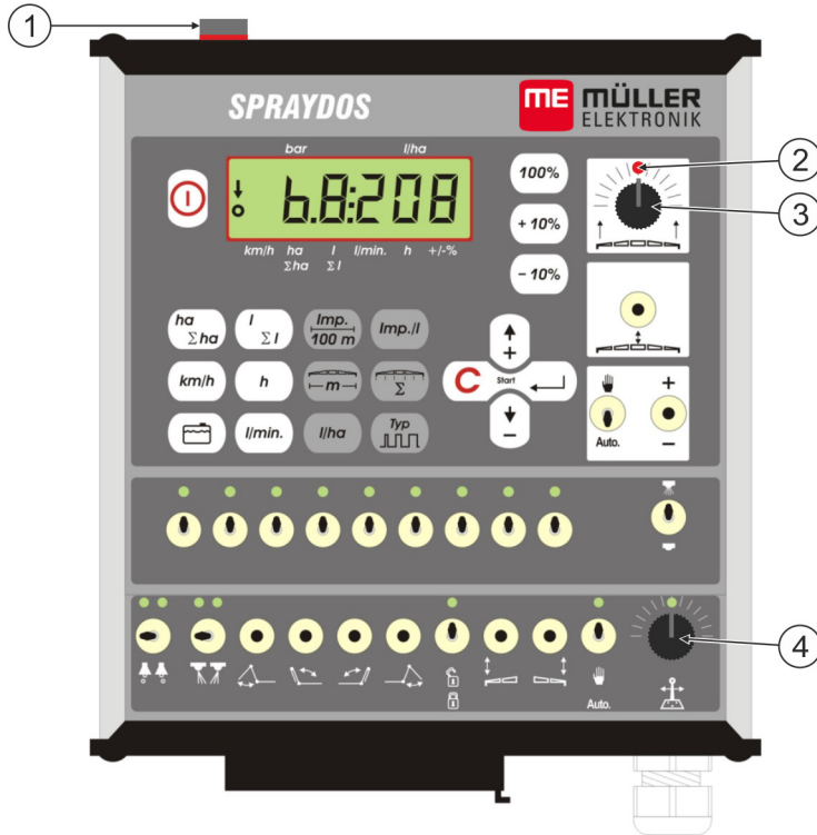
Рис. 6-3 Эксплуатационные элементы, необходимые для калибровки
